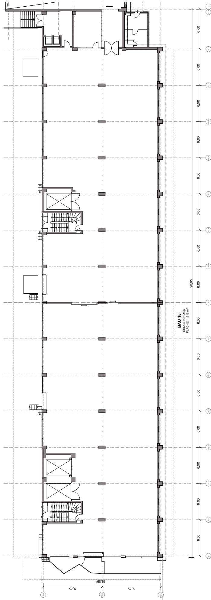
Bau 18 Grundriss Erdgeschoss
